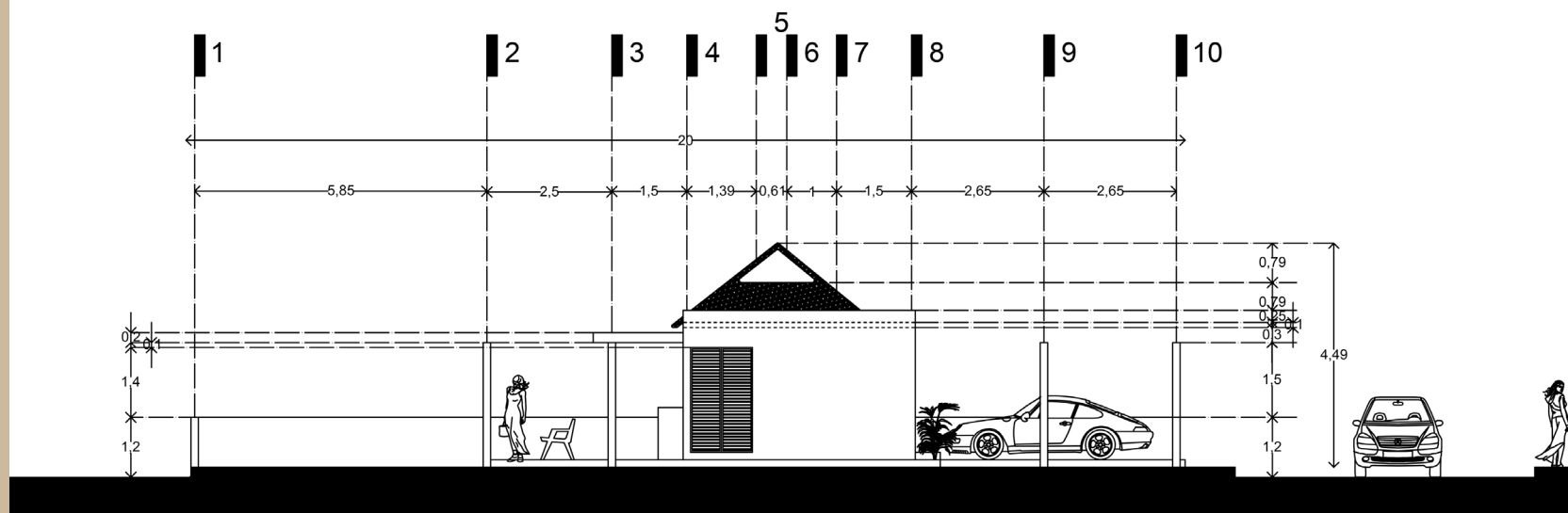
FACHADA IZQUIERDA
