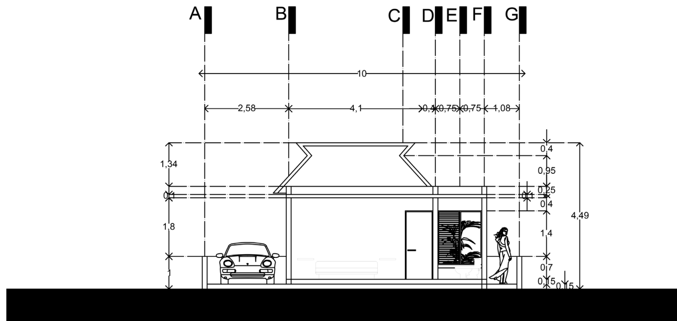
CORTE x1-x1
