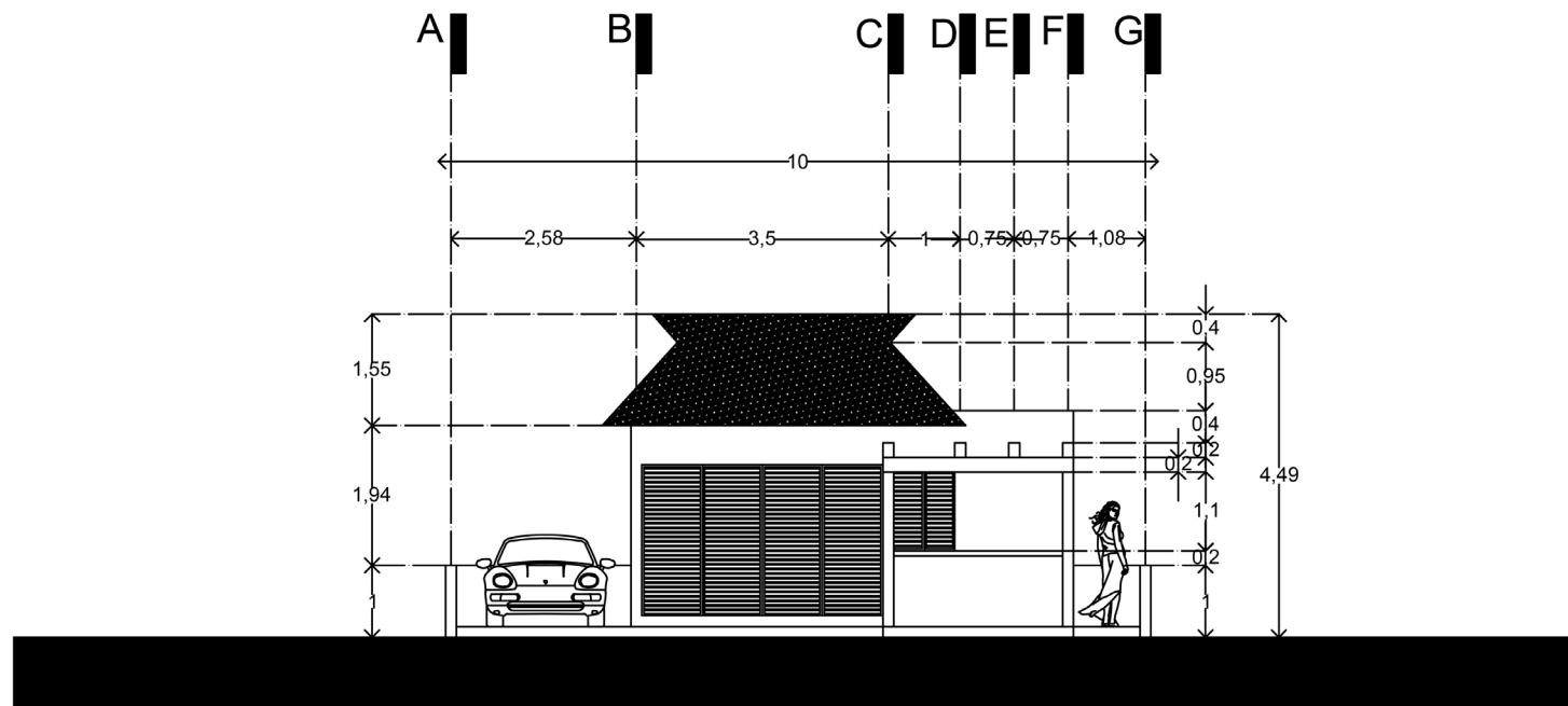
FACHADA TRASERA
